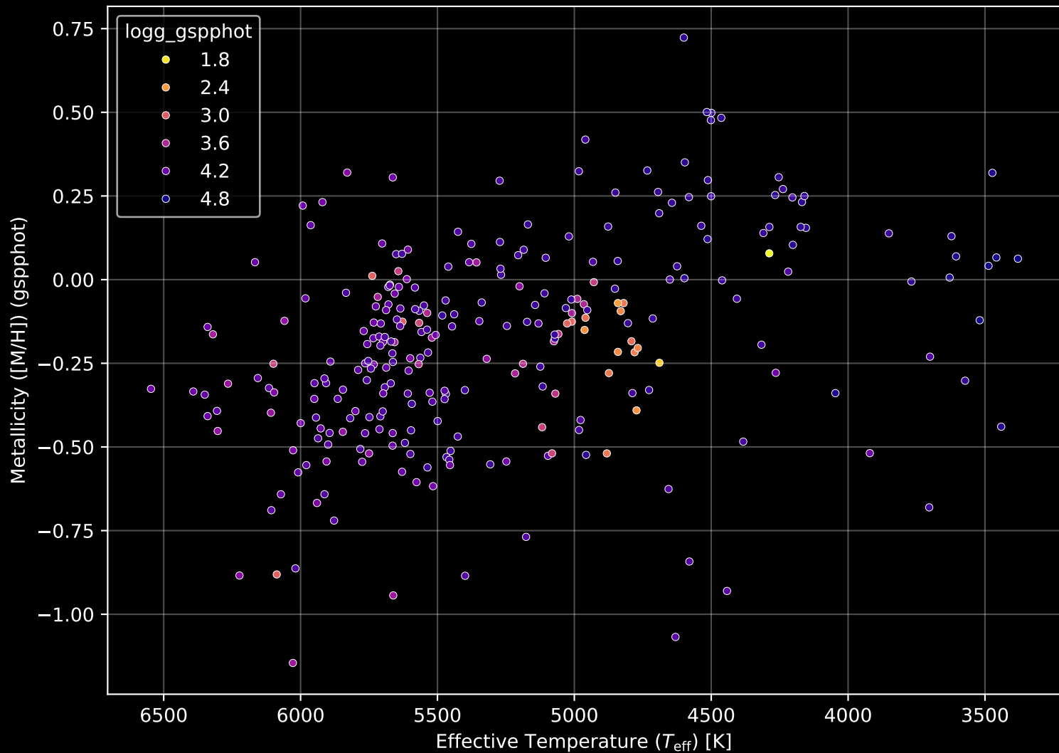
APOGEE DR17 Field: [sgr_tidal6] Stellar Population Parameters (n= 277)
